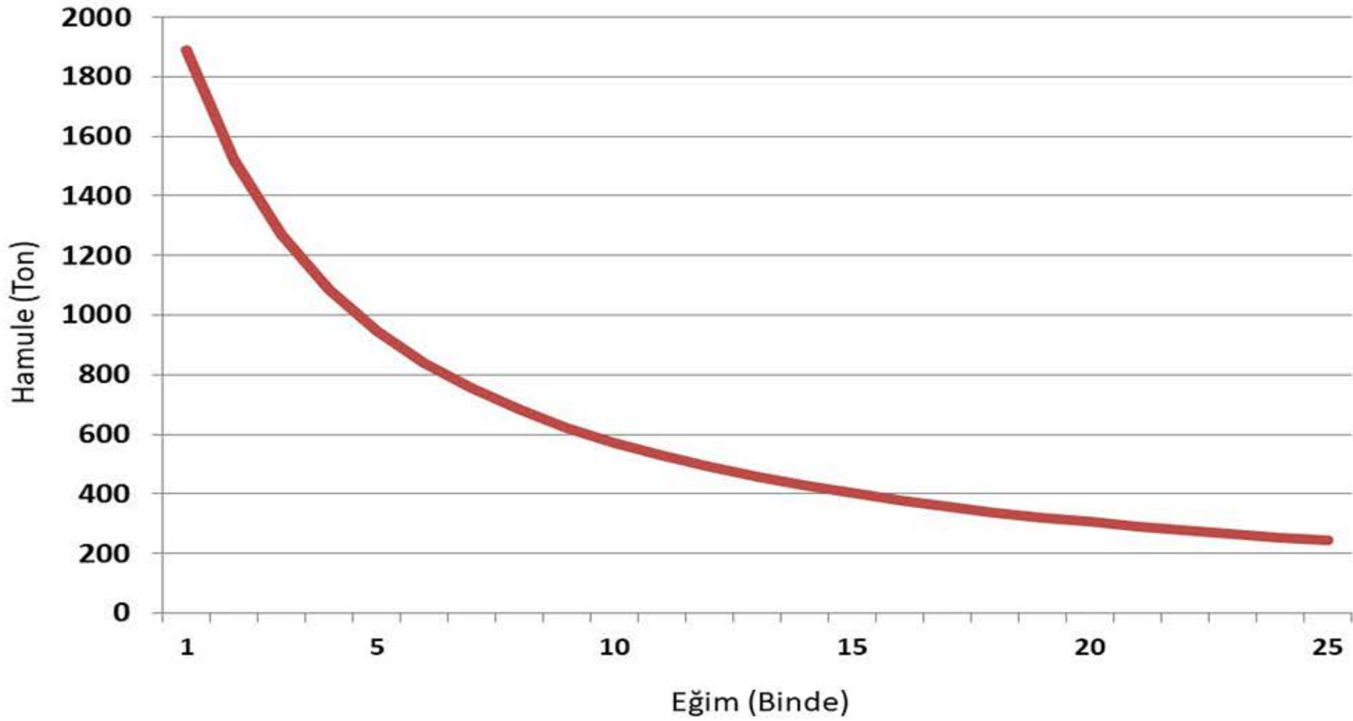
LDH 45 186 Tipi Dizel Hidrolik Lokomotifin Eğim Hamule Grafiği
